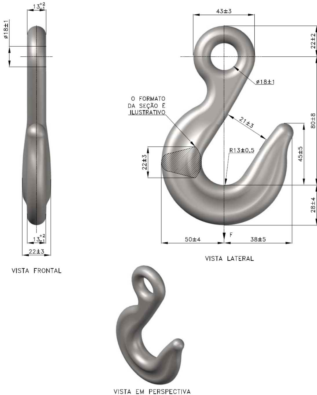
Figura 1 - Gancho Olhal
